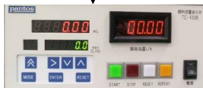
燃料流量表示計 TC-100B シリーズ 外形寸法 : W220×H99×D200
