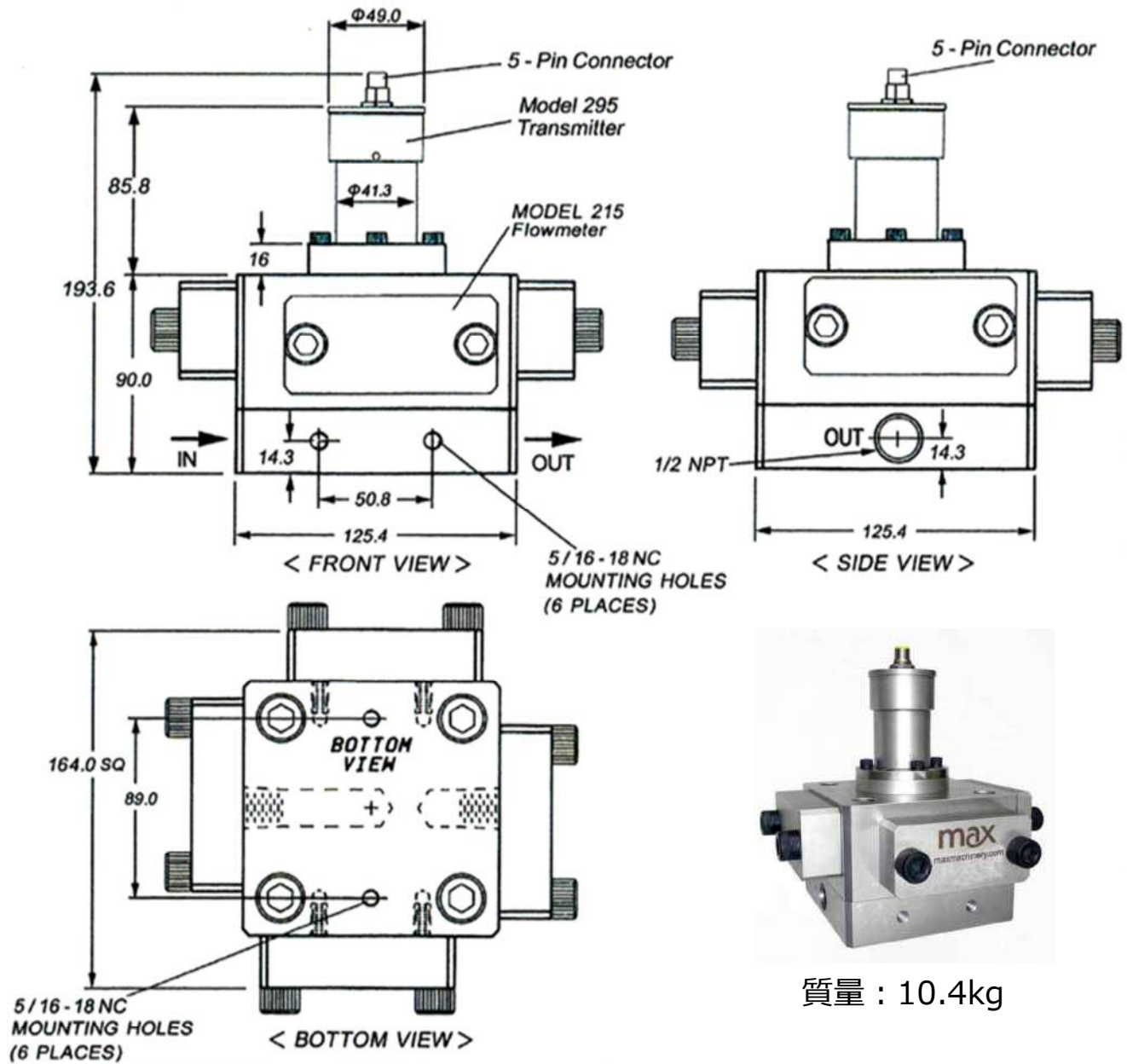
■ 型式 215/295F 流量計外形寸法図
