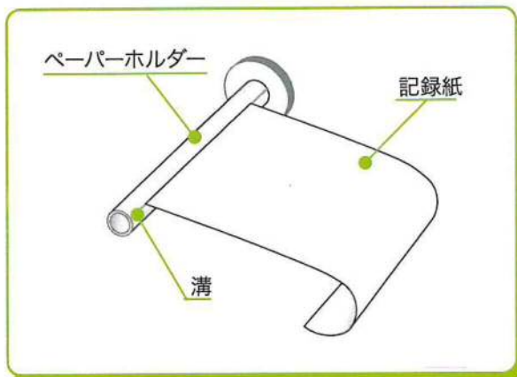
ペーパーホルダー部拡大図
